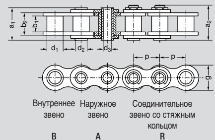
Тип А - втулочная цепь
