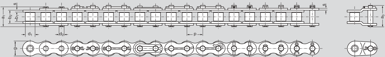
Внутреннее звено Наружное звено Наружное звено Наружное звено Соединительное звено со штифтом с тавровой головкой Наружное звено Соединительное звено со шплинтом Изогнутое звено со шплинтом В А AS AT Н АК U L
